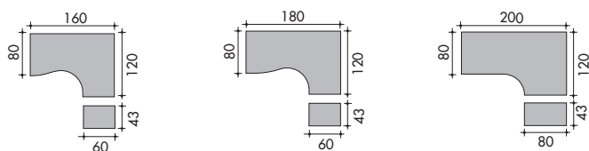
Асимметричные компактные столы
