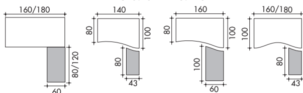
Приставные элементы для прямых, асимметричных компактных столов и столов "Волна"
